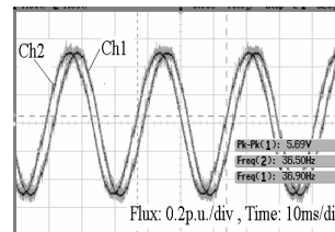
Fig.23.Ch1: \Psi_{s\alpha 1} Ch2: \Psi_{s\alpha 2}
