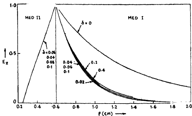
FIG. 8 (d). E_z vs \rho for \epsilon^0 = 1.062 .
